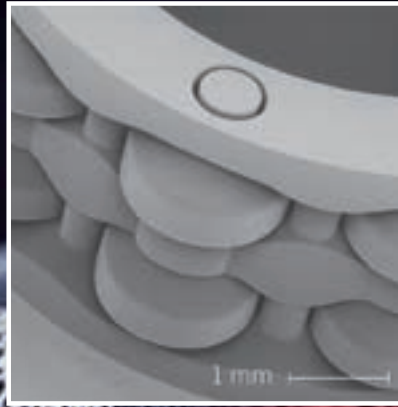
3D-Druck Nano Rollenlager
